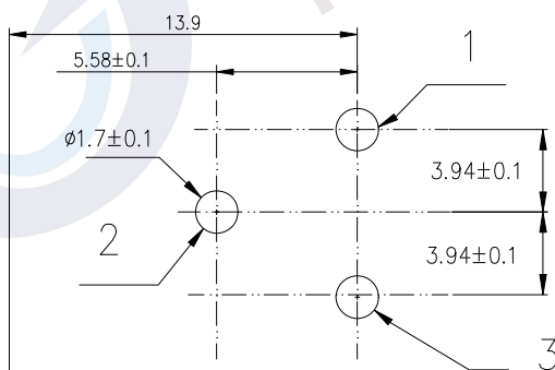
PCB板开孔尺寸图
