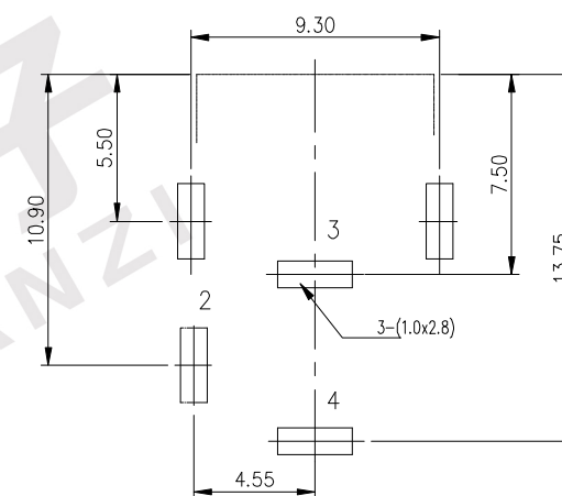
线路板开孔尺寸图
